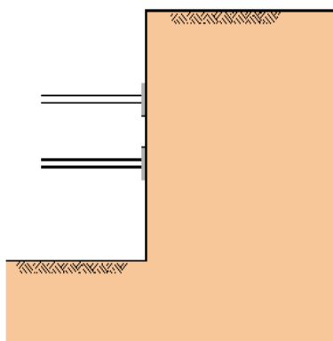
با کمک عنصرهای فشاری
