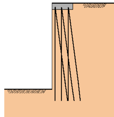
با کمک ریزشمع ها
